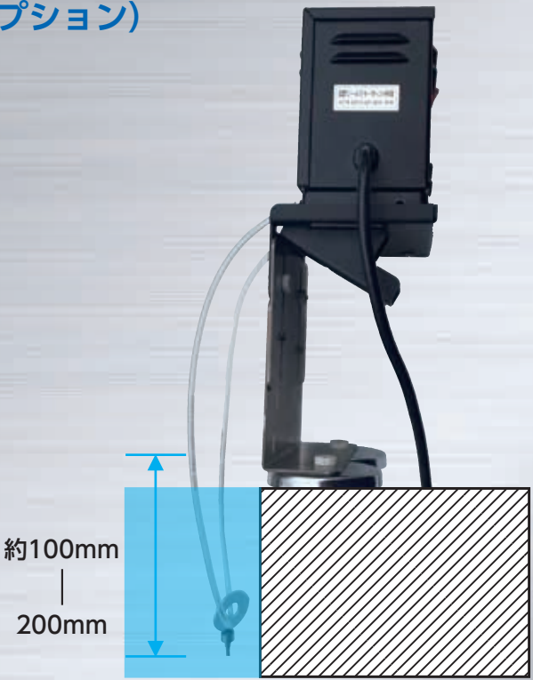
上面取付例
